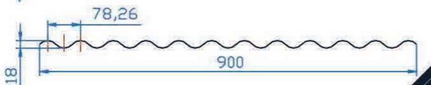
Tôle ondulée Corrugated sheet
